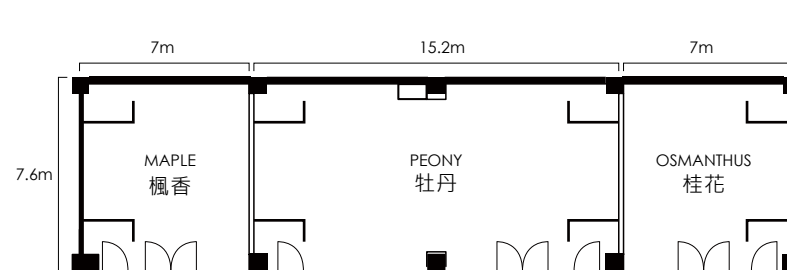
MULTI-FUNCTION ROOMS 多功能包廂平面圖
